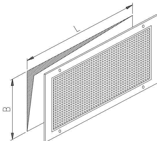
CNP perforált lemezes rács
