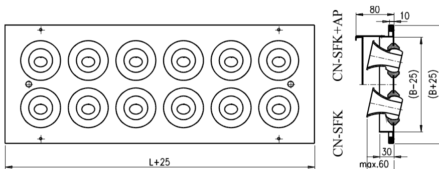
CN-SFK befűvó
